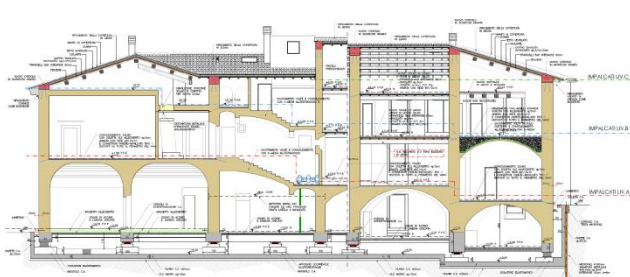
Figura 3: Intervento di isolamento sismico alla base di un aggregato in muratura nel centro storico di L'Aquila
